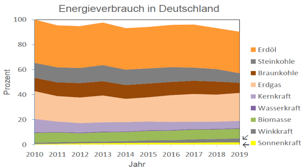
Abb. 2. Die Anteile der verschiedenen Energieträger an der gesamten (primären) Energieversorgung. Die Gesamtenergie im Jahr 2010 wurde auf 100% gesetzt. Quelle: BMWi.
